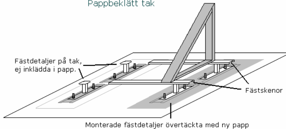
Pappbeklätt tak
